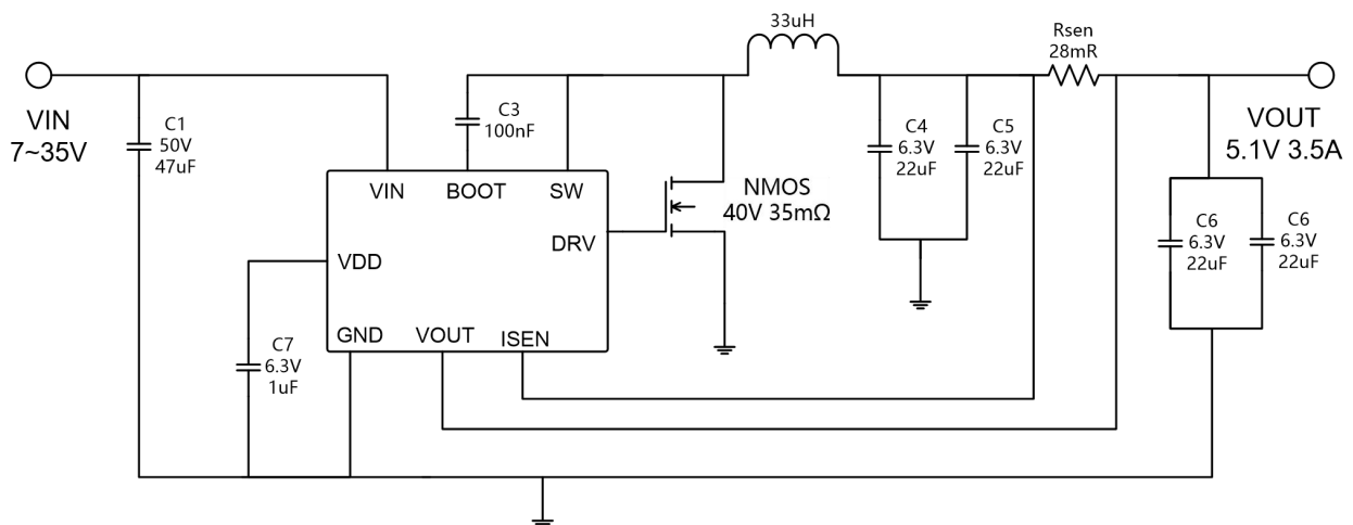
图 1 同步降压模式应用线路图
