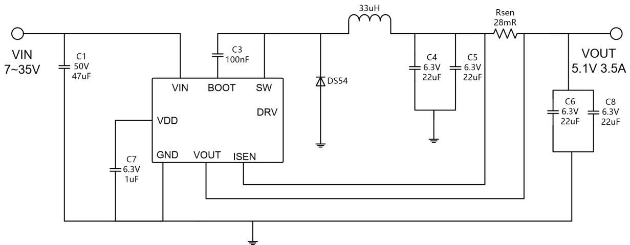
图 2 非同步降压模式应用线路图
