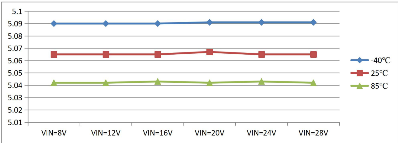
输出调整率测试
