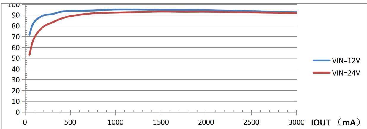
恒流测试VIN=12V/24V Rsen=33mΩ
